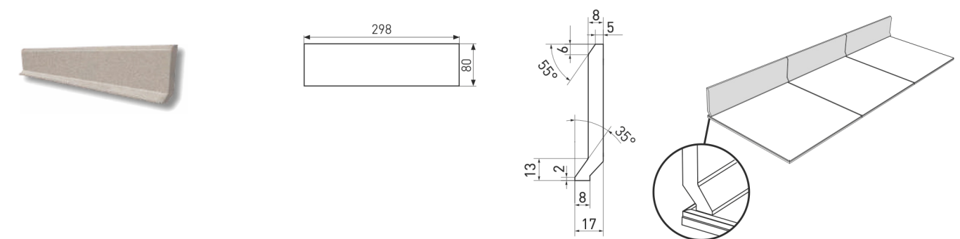
SOKKELHULKEHL - 80x298x8 mm - (TSFKF0..) - vinklet top
